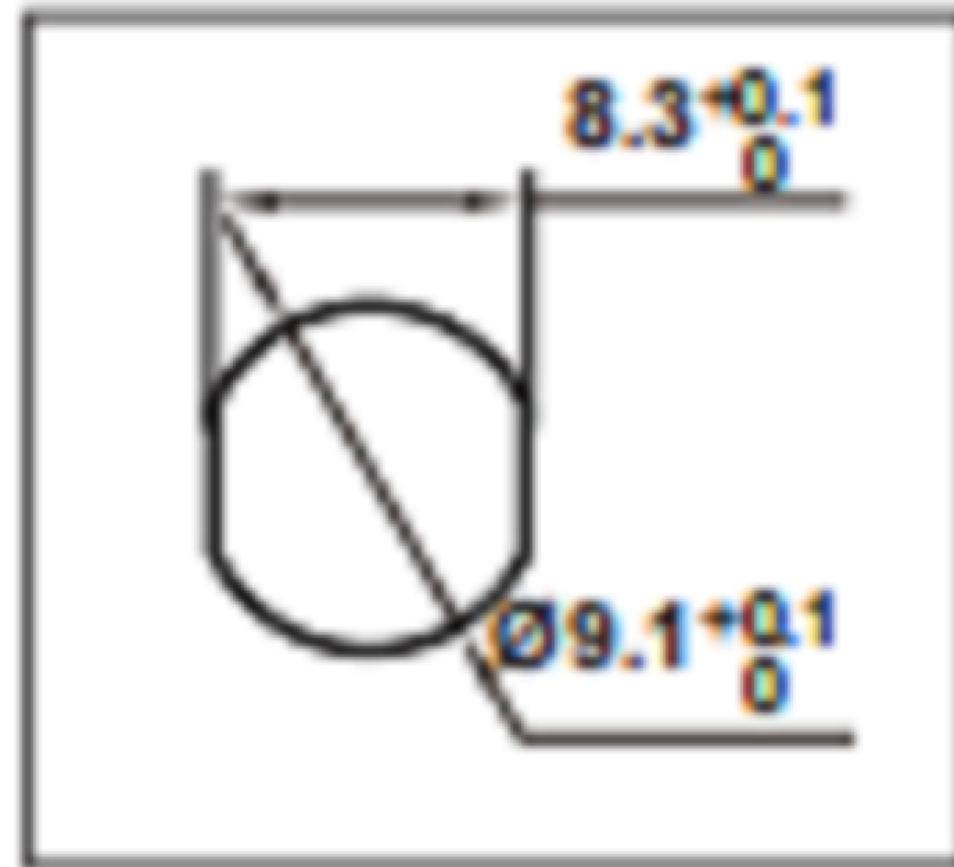
面板开孔图
